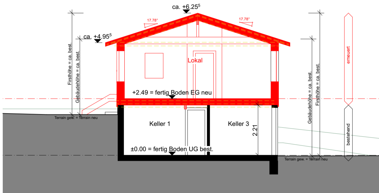
Schnitt 3-3
