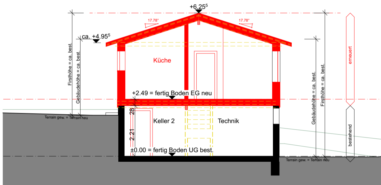
Schnitt 2-2
