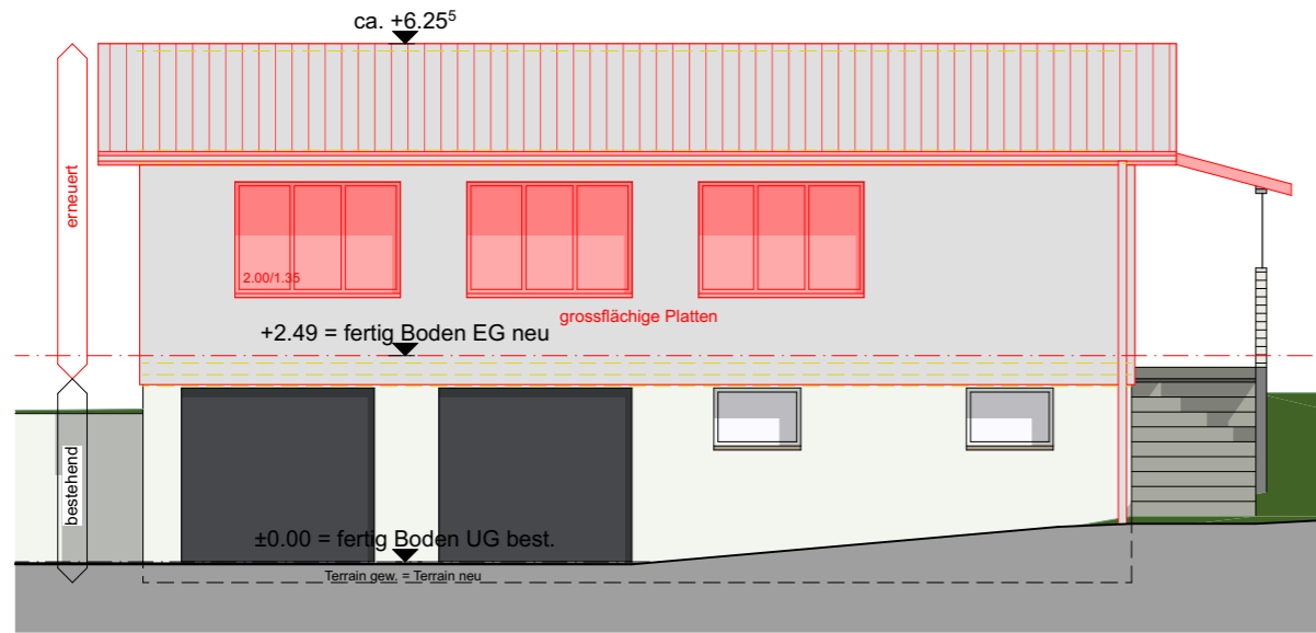
Südfassade
